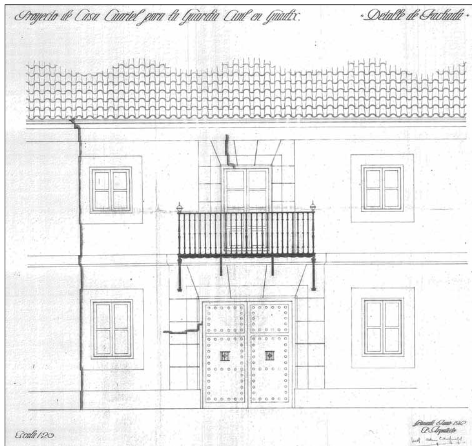
Fig.2. Detalle de fachada del Cuartel de la Guardia Civil.
