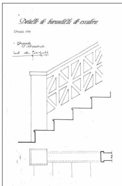
Figs.4 y 5. Detalles de barandilla de escalera y mirilla.
