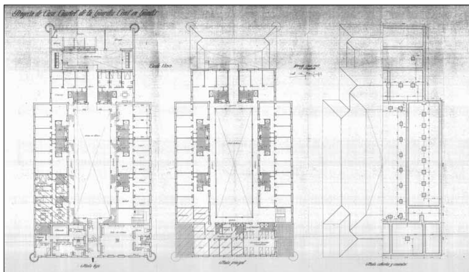
Fig.6. Plano del edificio del Cuartel de la Guardia Civil de Guadix, construido por Regiones Devastadas.
