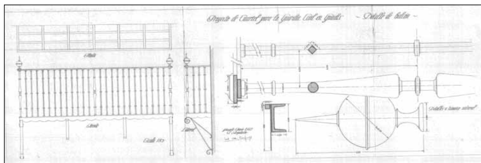
Fig.3. Detalles del Balcón de la Fachada del Cuartel de la Guardia Civil.
